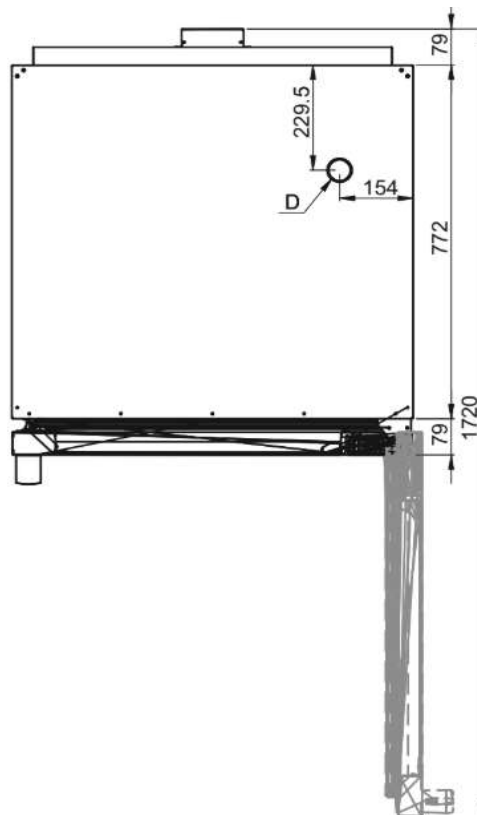
Vue d'en haut porte ouverte
