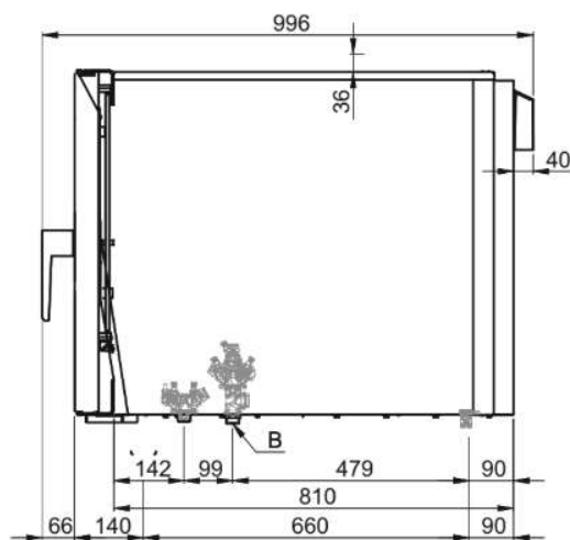
Vue côté
